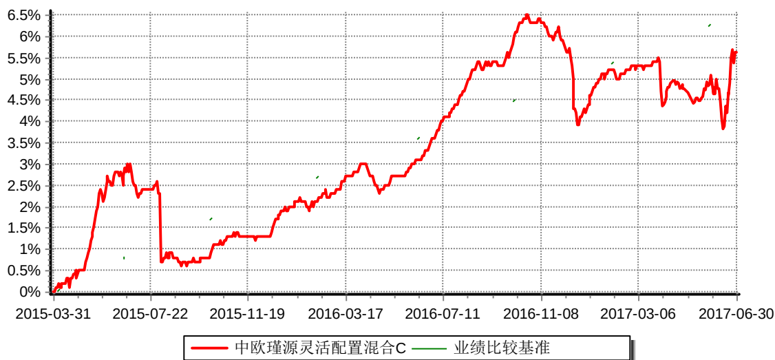
中欧瑾源灵活配置混合C 累计净值增长率与业绩比较基准收益率历史走势对比图 (2015年03月31日-2017年06月30日)
